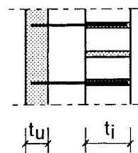
Ingjutna respektive innmurade kramlor
